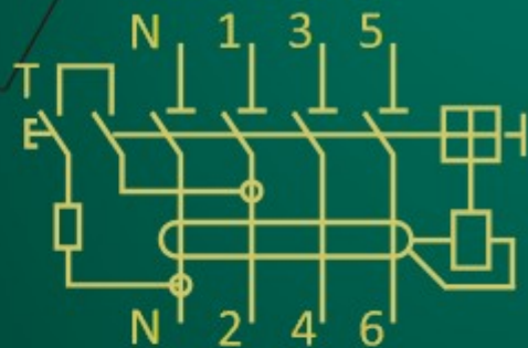
دیاگرام فنی (چهارپل)
